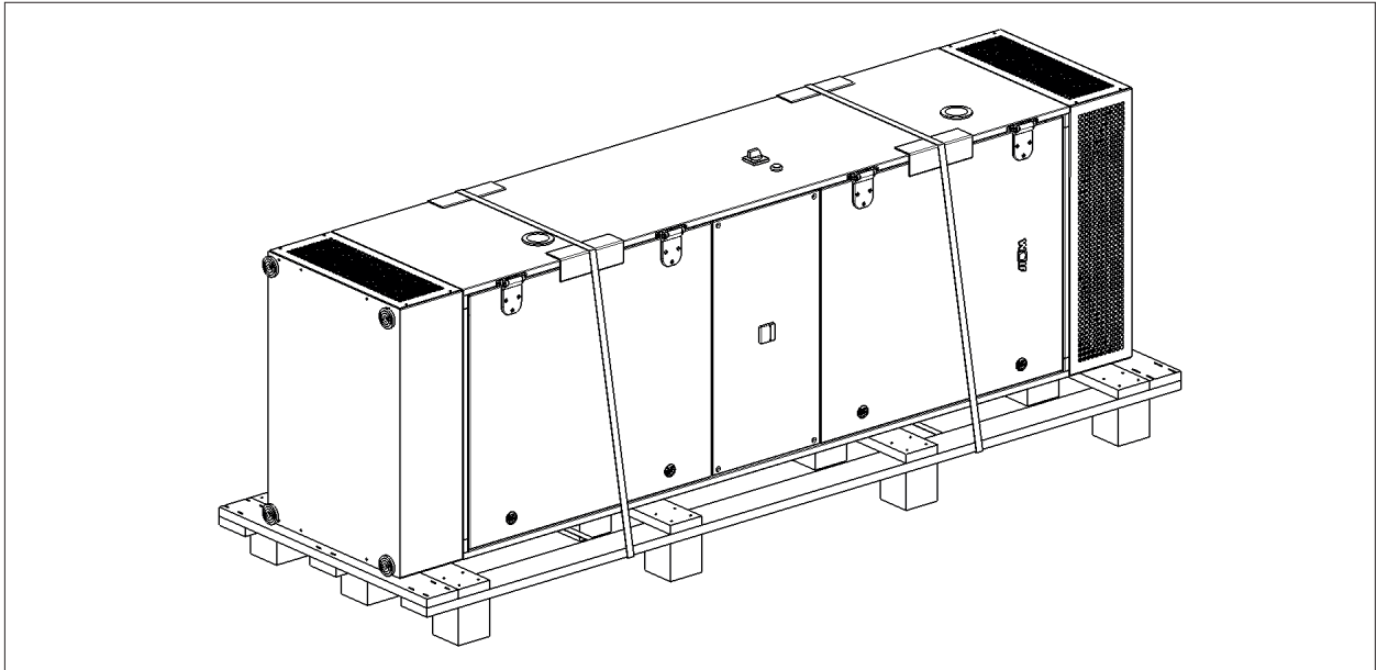
Abb. 4.1 Auslieferungszustand
